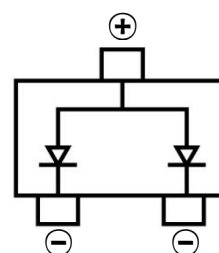
SOT-23
