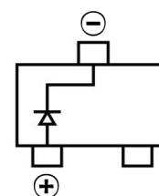
BAS21:JS
