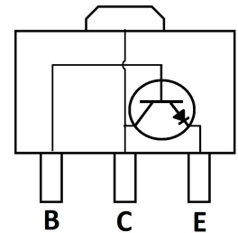
SOT-89
