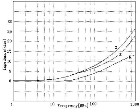
HDGB2012M260HT-LF
