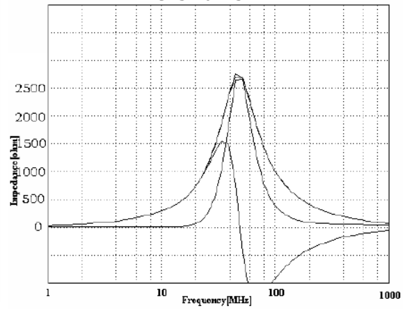
HDGB3216M252HT-LF
