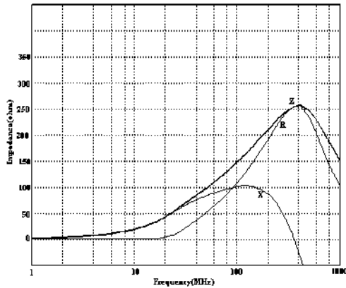
HDGB2012M151HT-LF
