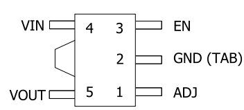
SOT-89-5L
