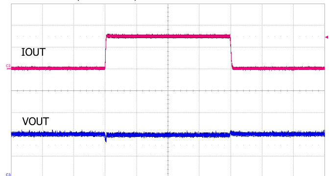
IOUT : 2.0A/div, VOUT : 100mV/div, Time : 500µs/div Load Transient Response
