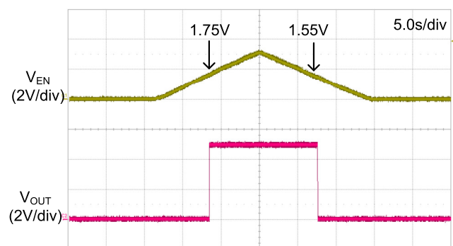
Enable Threshold
