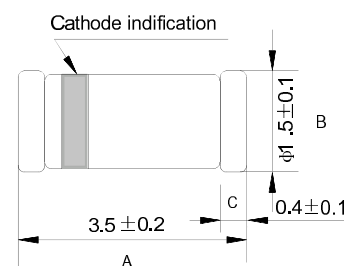
LL34 (SOD-80)
